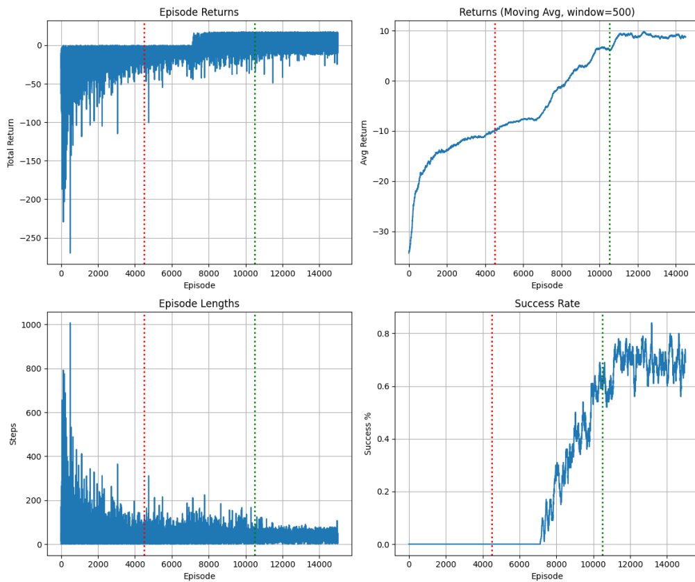
Figura 4: Métricas de entrenamiento en Entorno 2: retornos, media móvil, longitud de episodios y tasa de éxito.
